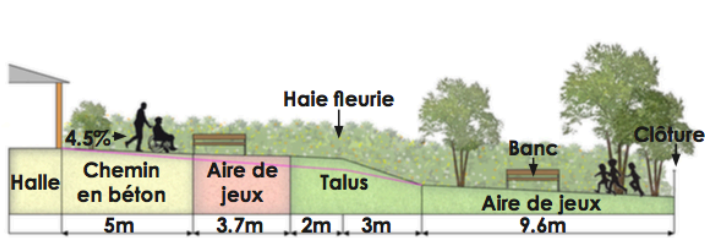
Coupe de principe AA' - projet
