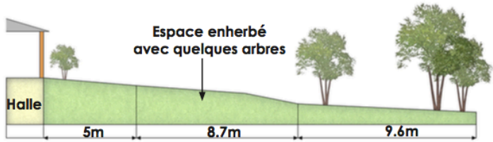
Coupe de principe AA' - état initial
