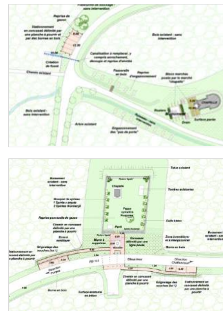
Plans techniques par village Phase DCE
